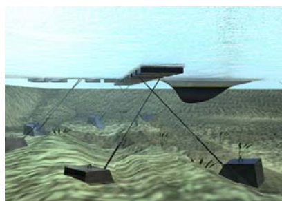
Seaflex forankringssystem
